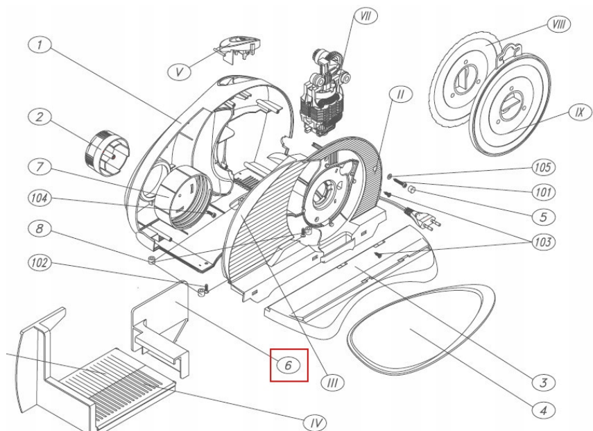
6 - Dociskacz 293.0002 - 1 sztuka
